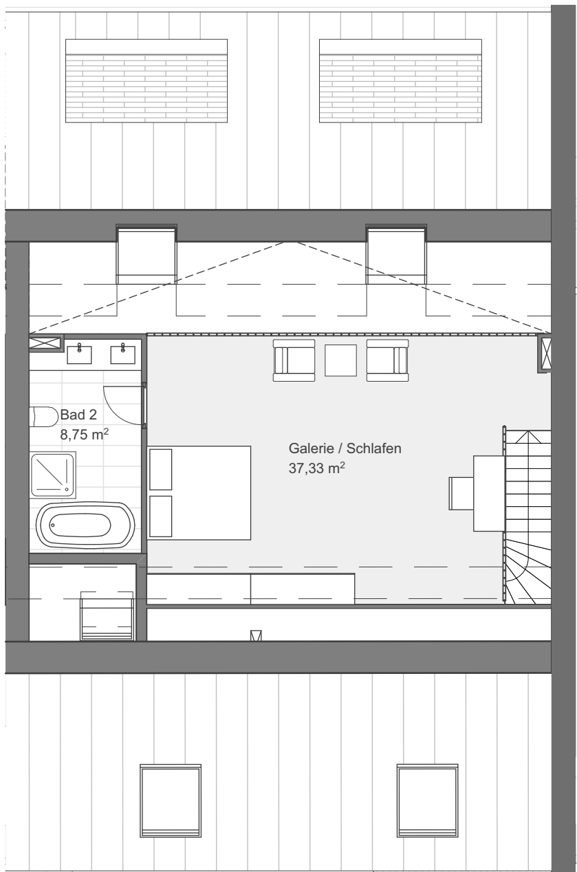
3. Obergeschoss
