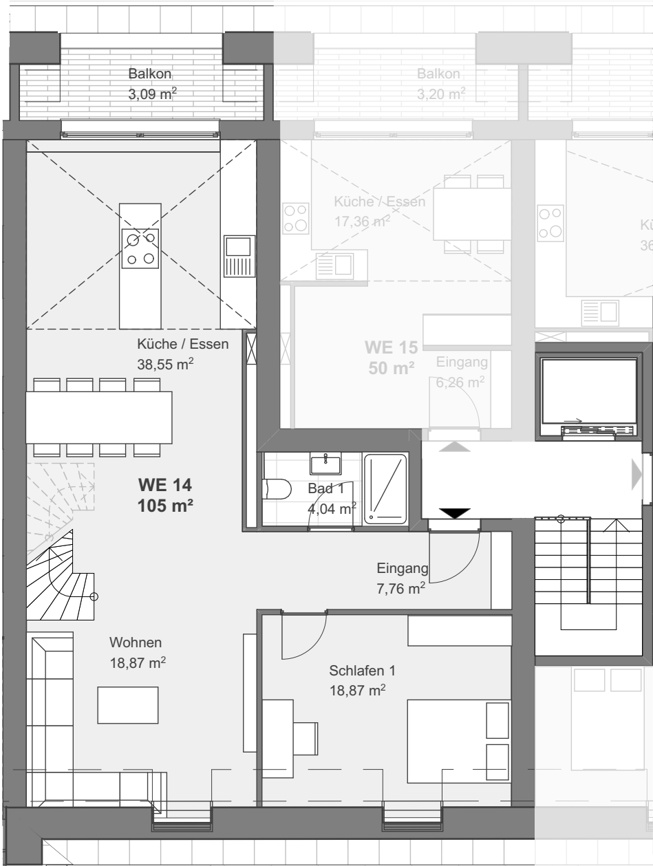
2. Obergeschoss
