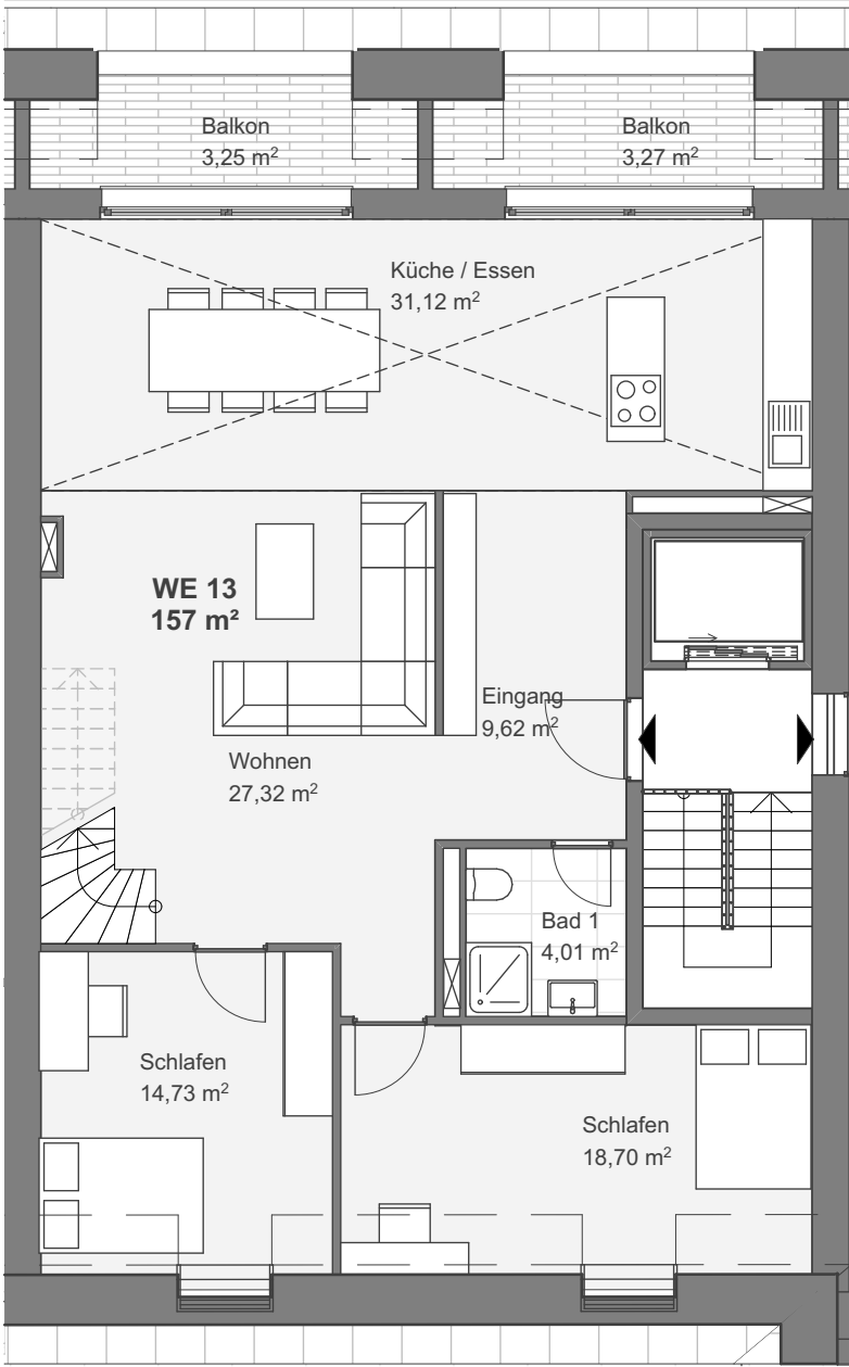
2. Obergeschoss
