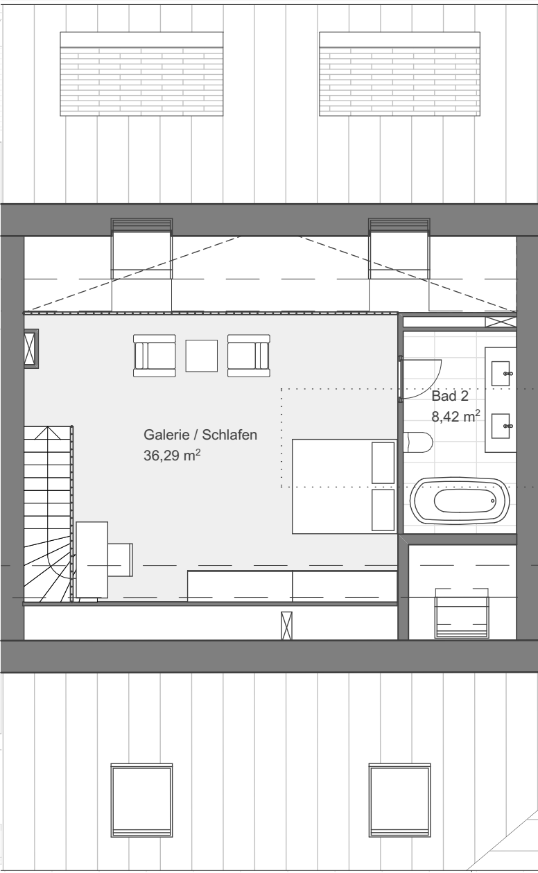
3. Obergeschoss
