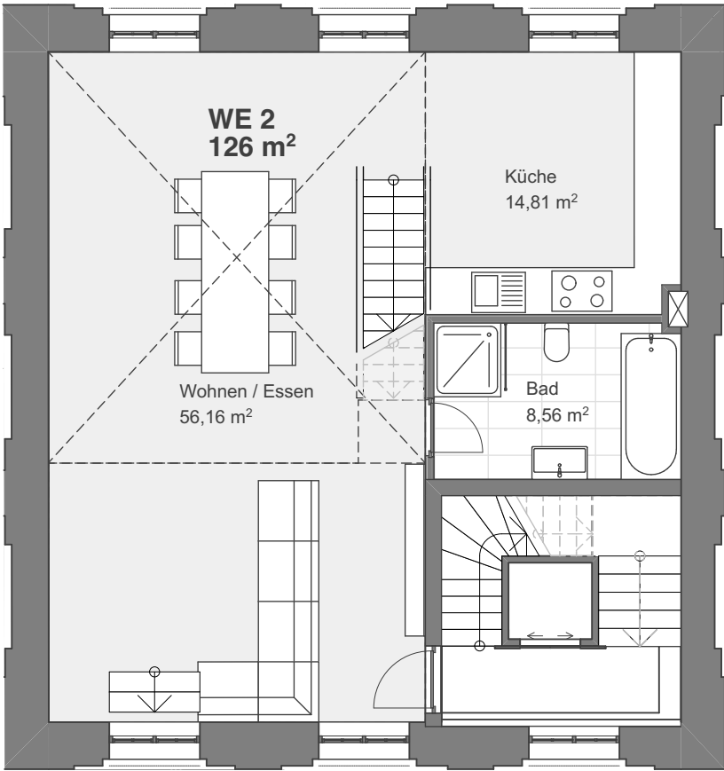
2. Obergeschoss
