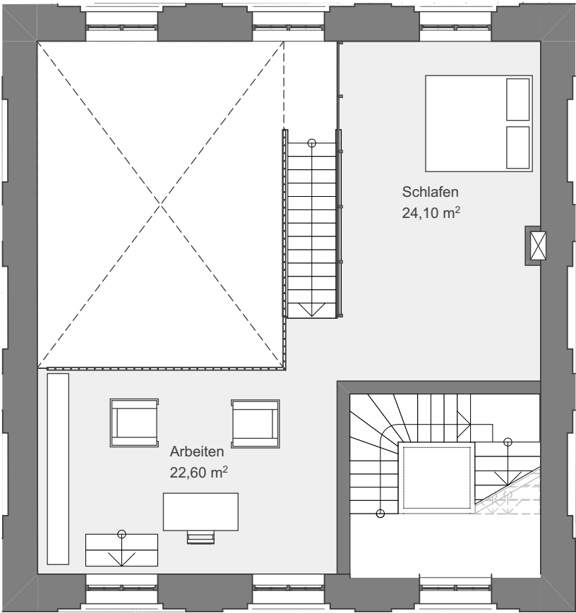
3. Obergeschoss
