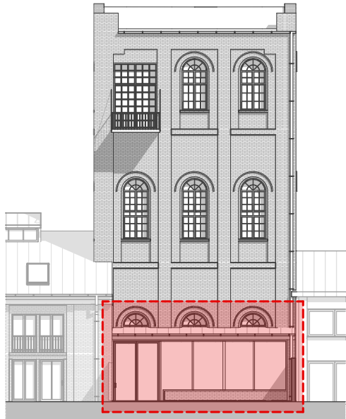
Süd Ansicht
